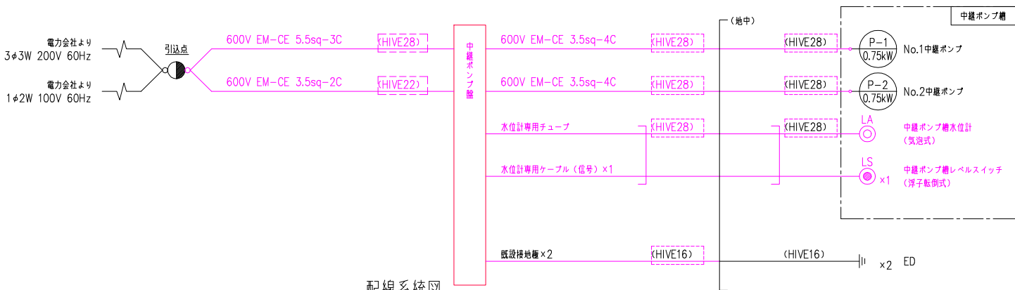
配線系統図
