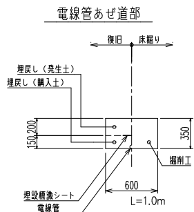
標準掘削断面図 S=1/30
