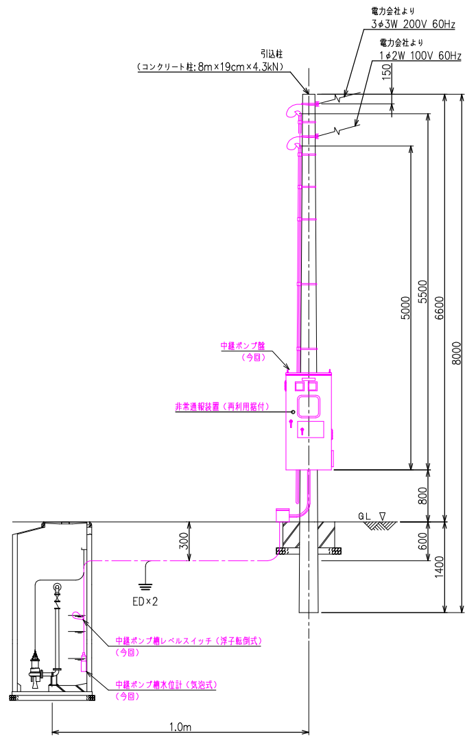
断面図 S=NON
