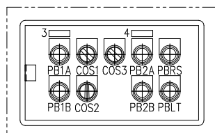
小扉部詳細 S=1/5
