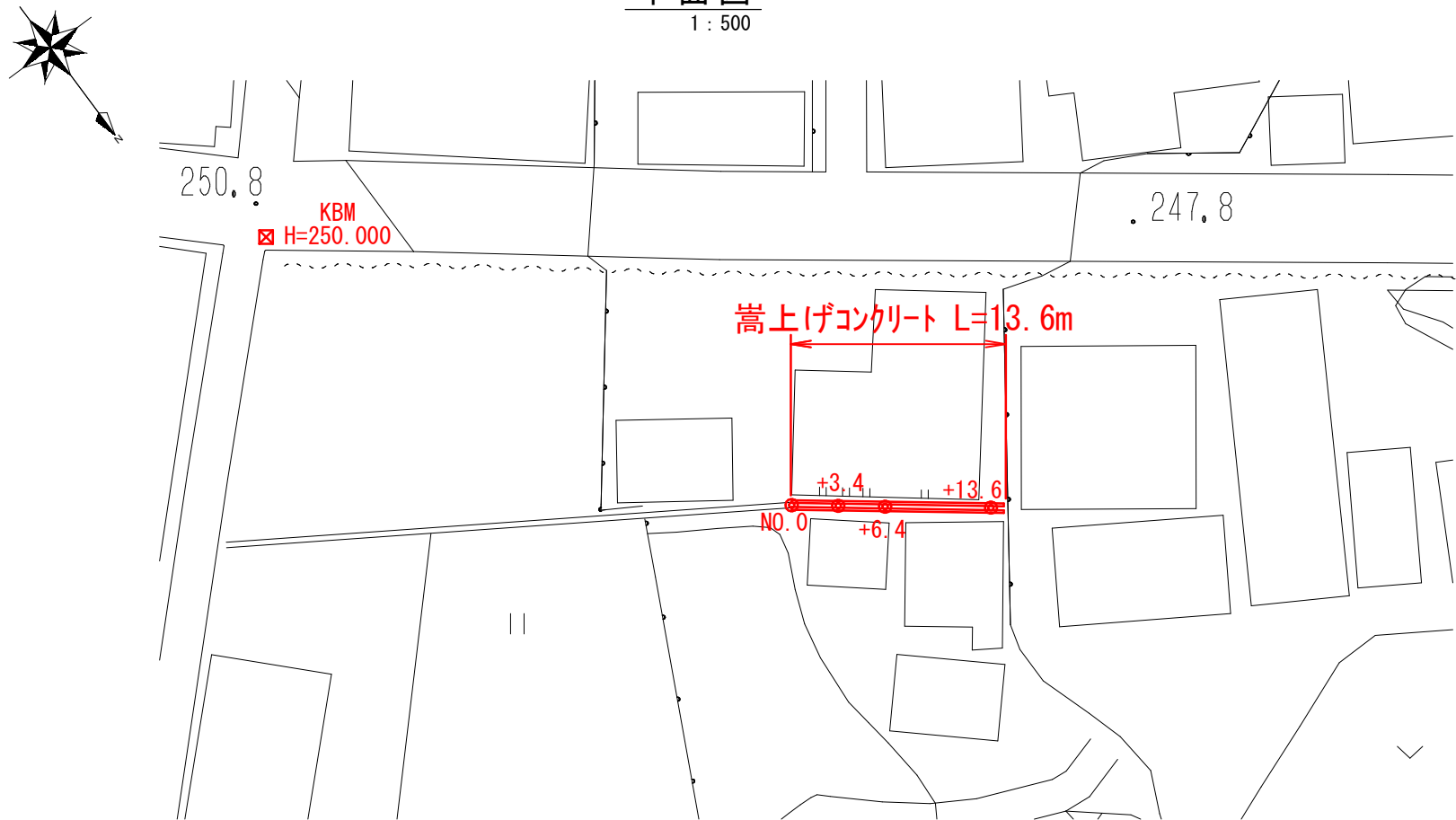
平面図
