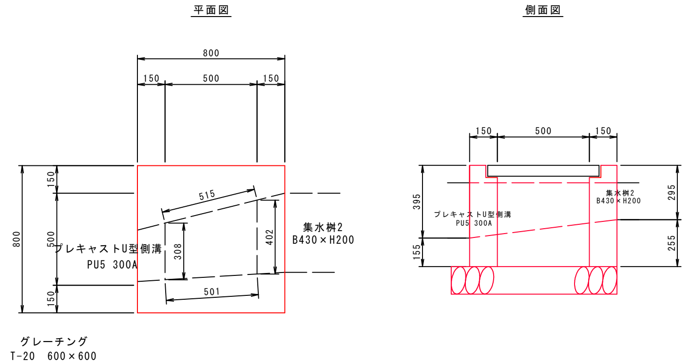
現場打ち水路
