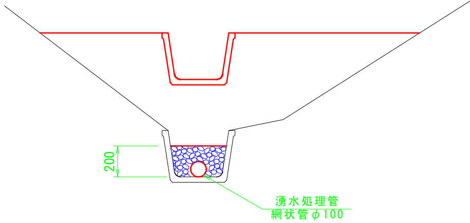
湧水処理工-1
