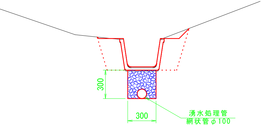
湧水処理工-2
