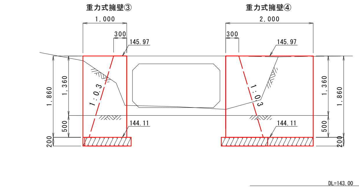
下流側側面図
