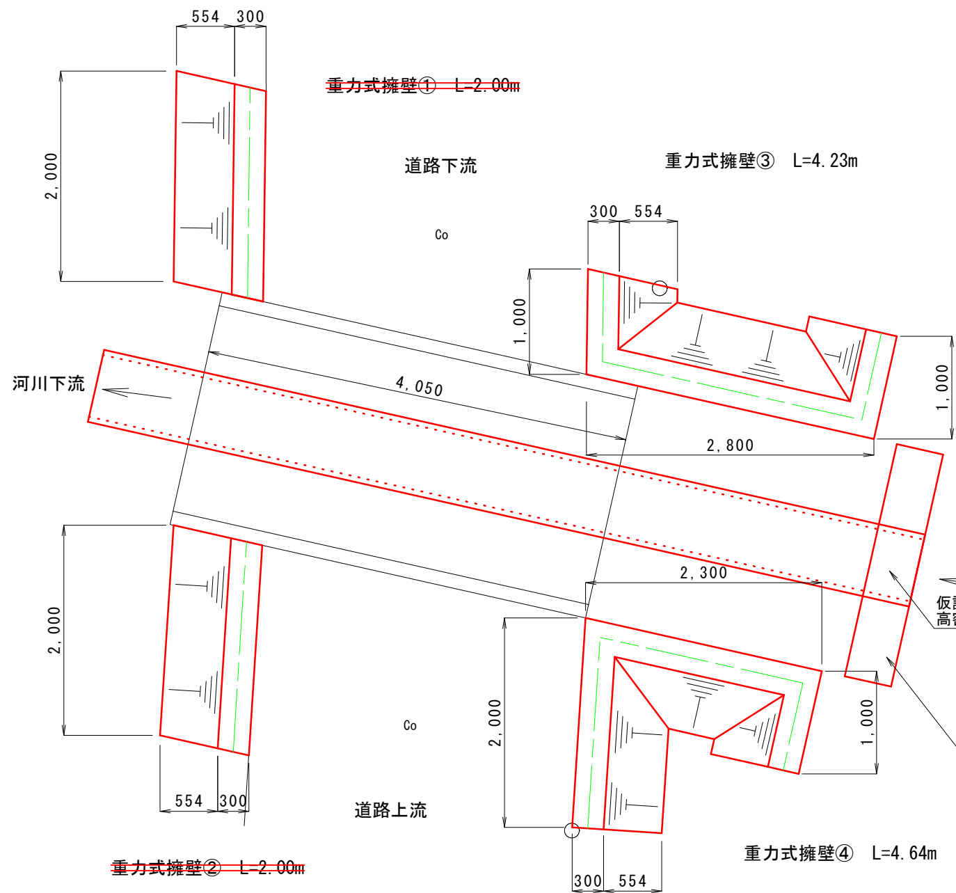
構造図 (SGW82) S=1:50
