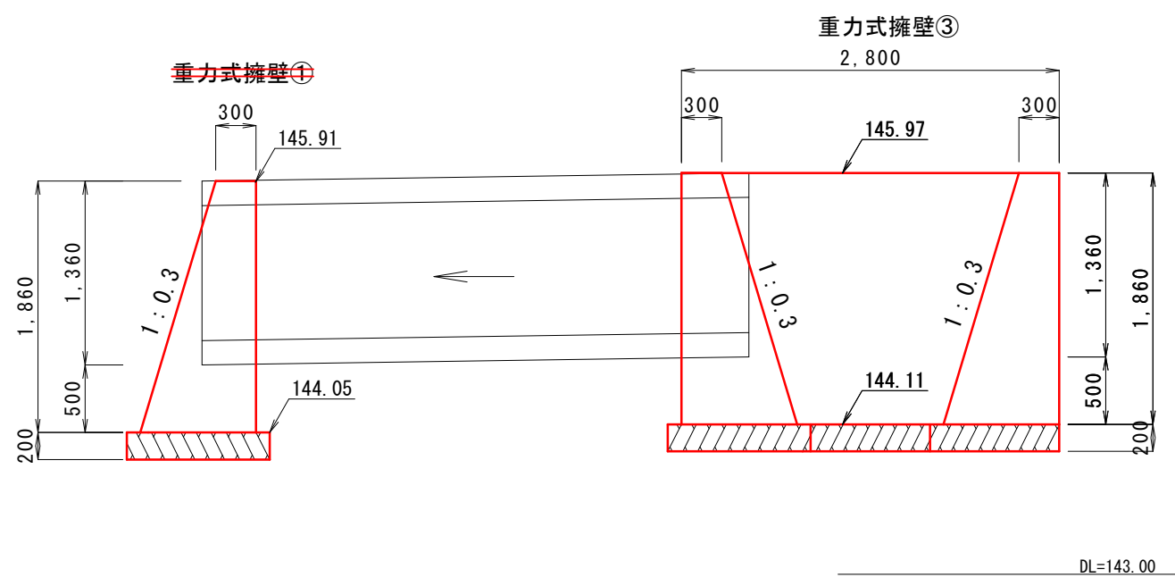
道路上流側断面図
