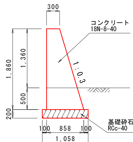
構造図 (SGW82) S=1:50
