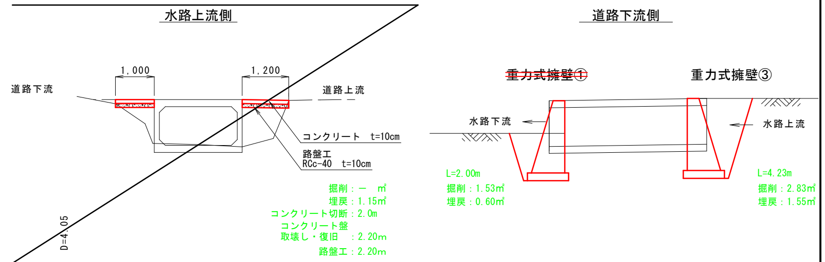
横断図 S=1:100
