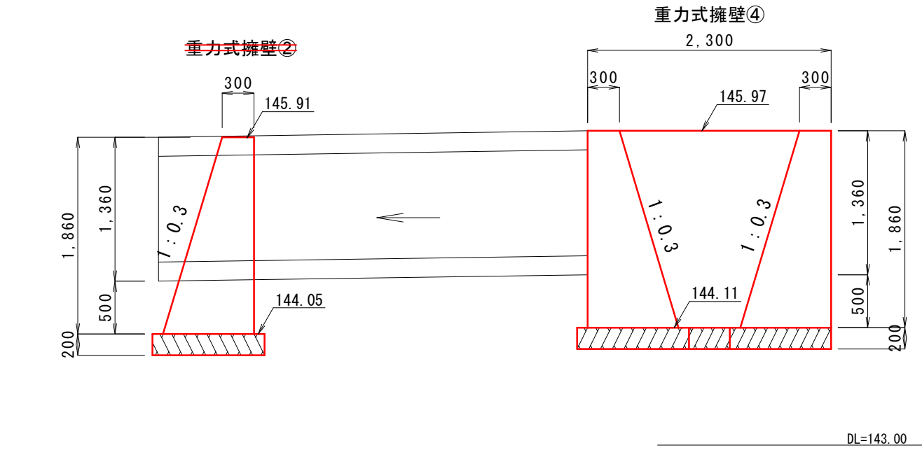
道路上流側断面図
