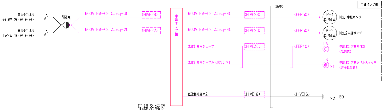
配線系統図
