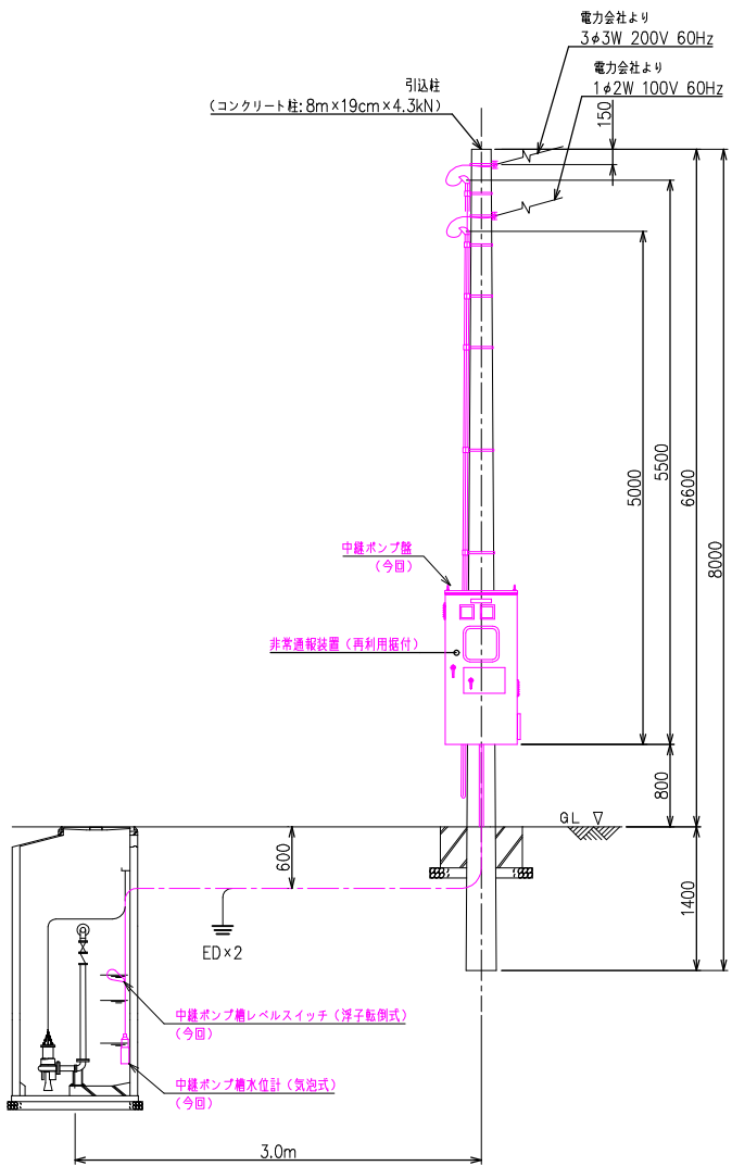
断面図 S=NON
