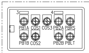
小扉部詳細 S=1/5
