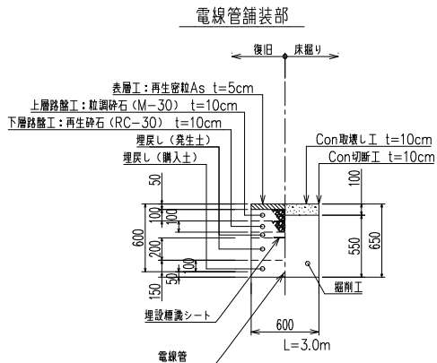
標準掘削断面図 S=1/30
