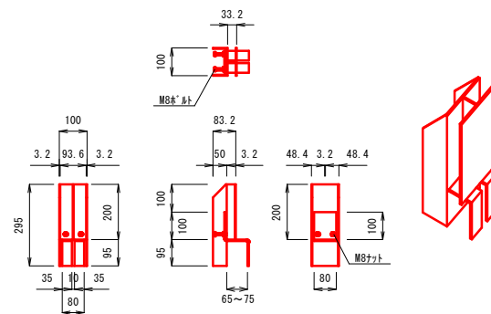
支間金具形状図 (参考図)
