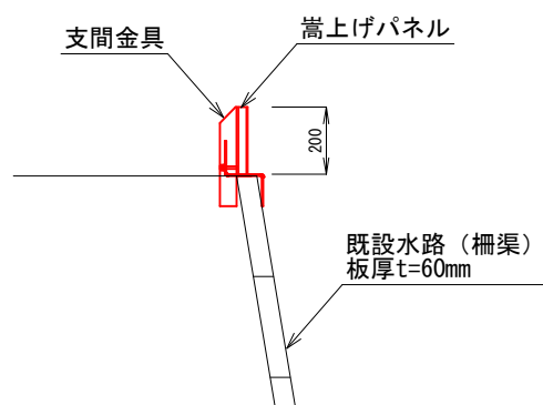
嵩上パネル断面図
